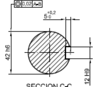
SECCION C-C
