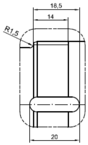
DETALLE W (2.5:1)
