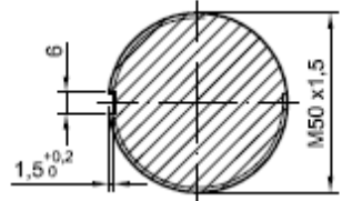
SECCION B-B
